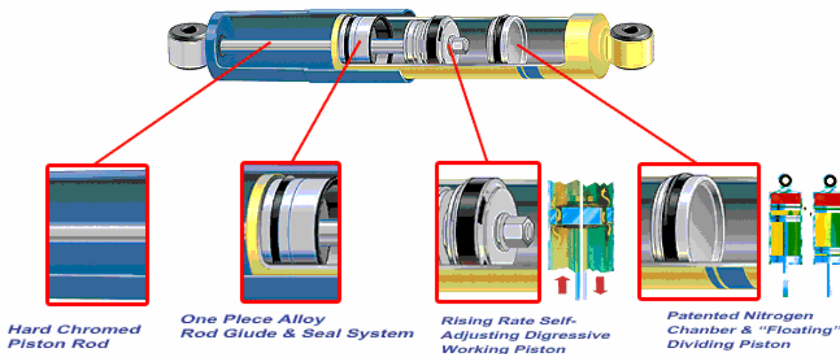
Obr. 2.3 Jednoplášťový plynokapalinový tlumič značky BILSTEIN [14]
