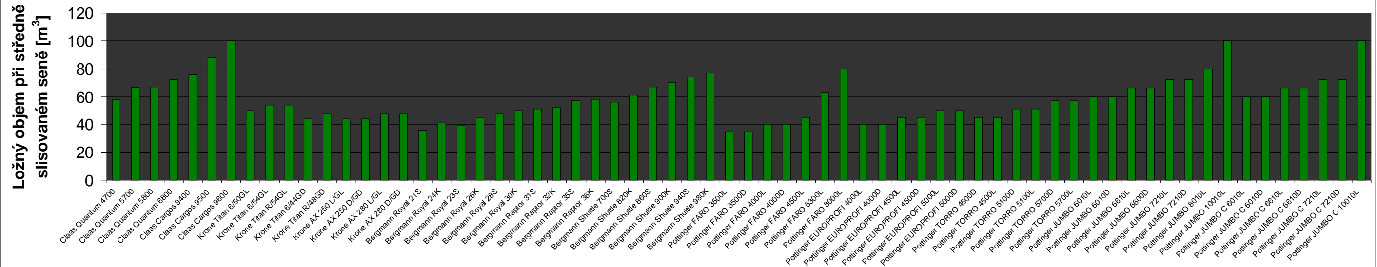
Srovnání samosběrných vozů podle ložného objemu při středně slisovaném seně
