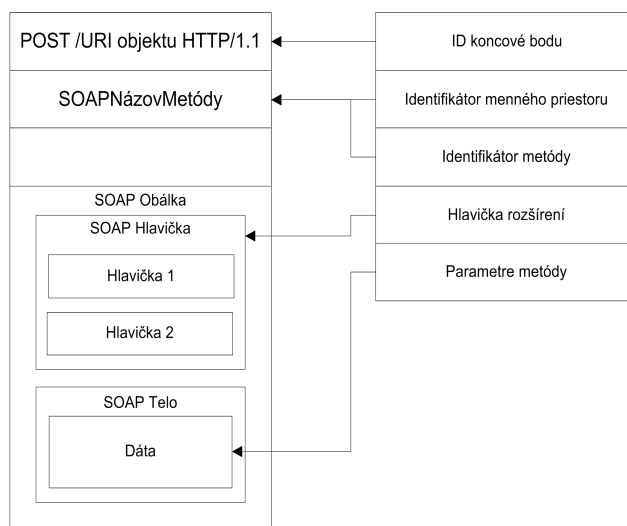
Obr. 2: Jednoduchá SOAP GET požiadavka
