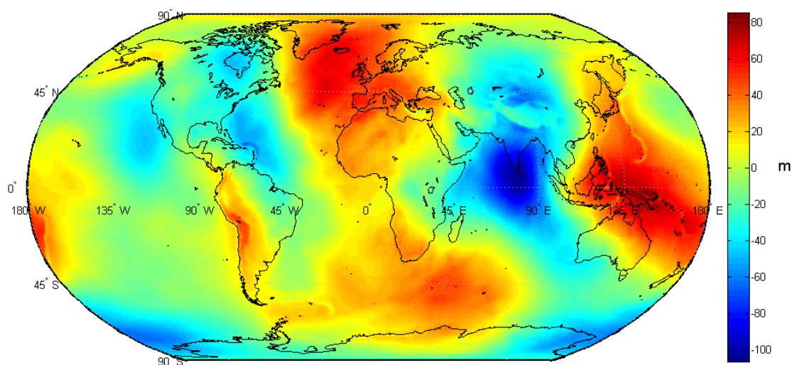
Obr. 1 vizualizace geoidu z modelu GOCE
