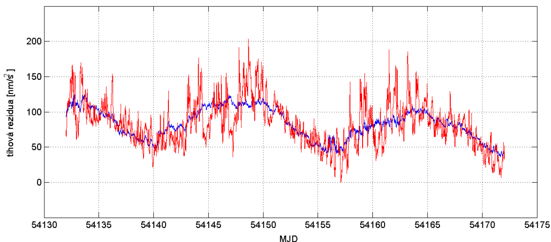
Obr. 3 původní signál tíhových reziduí (červeně) a signál opravený frekvenčně-závislou přenosovou funkcí (modře), datum je vyjádřeno pomocí modifikovaného Juliánského data (MJD)
