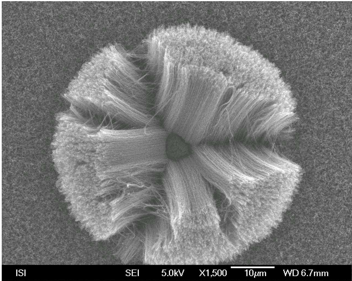
Obr. 2: SEM snímek uhlíkových nanotrubic
