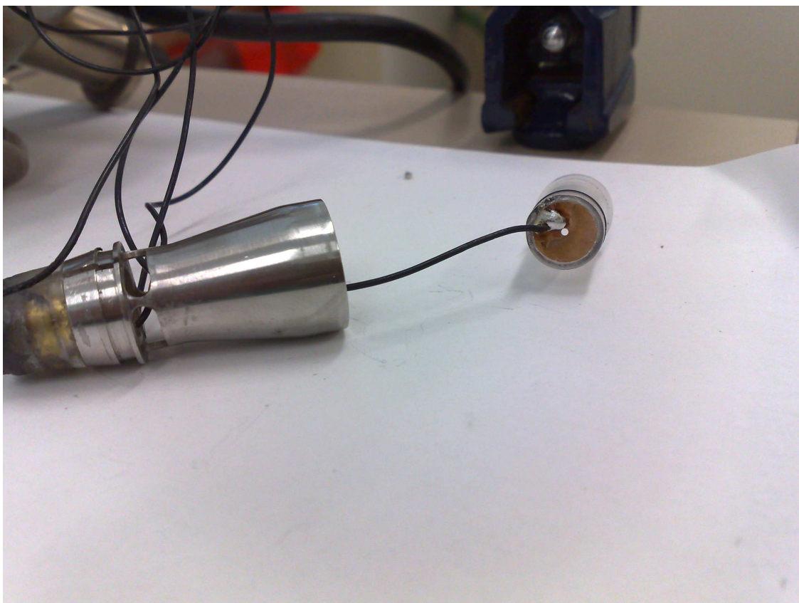
Obr.2 Ukázka připájené nové clonky C 2 o velikosti otvoru 1 mm.
