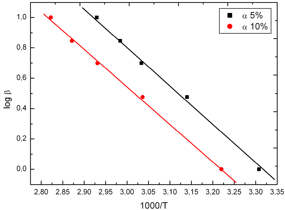
Obrázok č.14 priebeh závislosti \log \beta = f\left(\frac{1000}{T}\right) .
