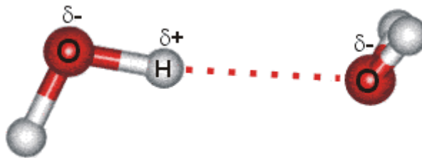
Obrázok č.6 Znázornenie vodíkového mostíka medzi dvomi molekulami vody [9].
