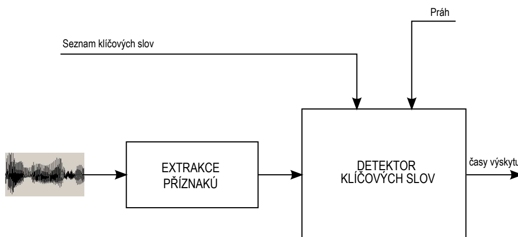
Obr. 2.1: Obecné schéma detektoru klíčových slov
