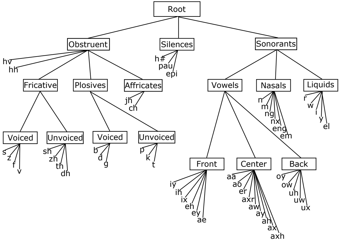
Obr. 3.1: Hierarchická fonémová struktura pro anglickou fonetickou abecedu
