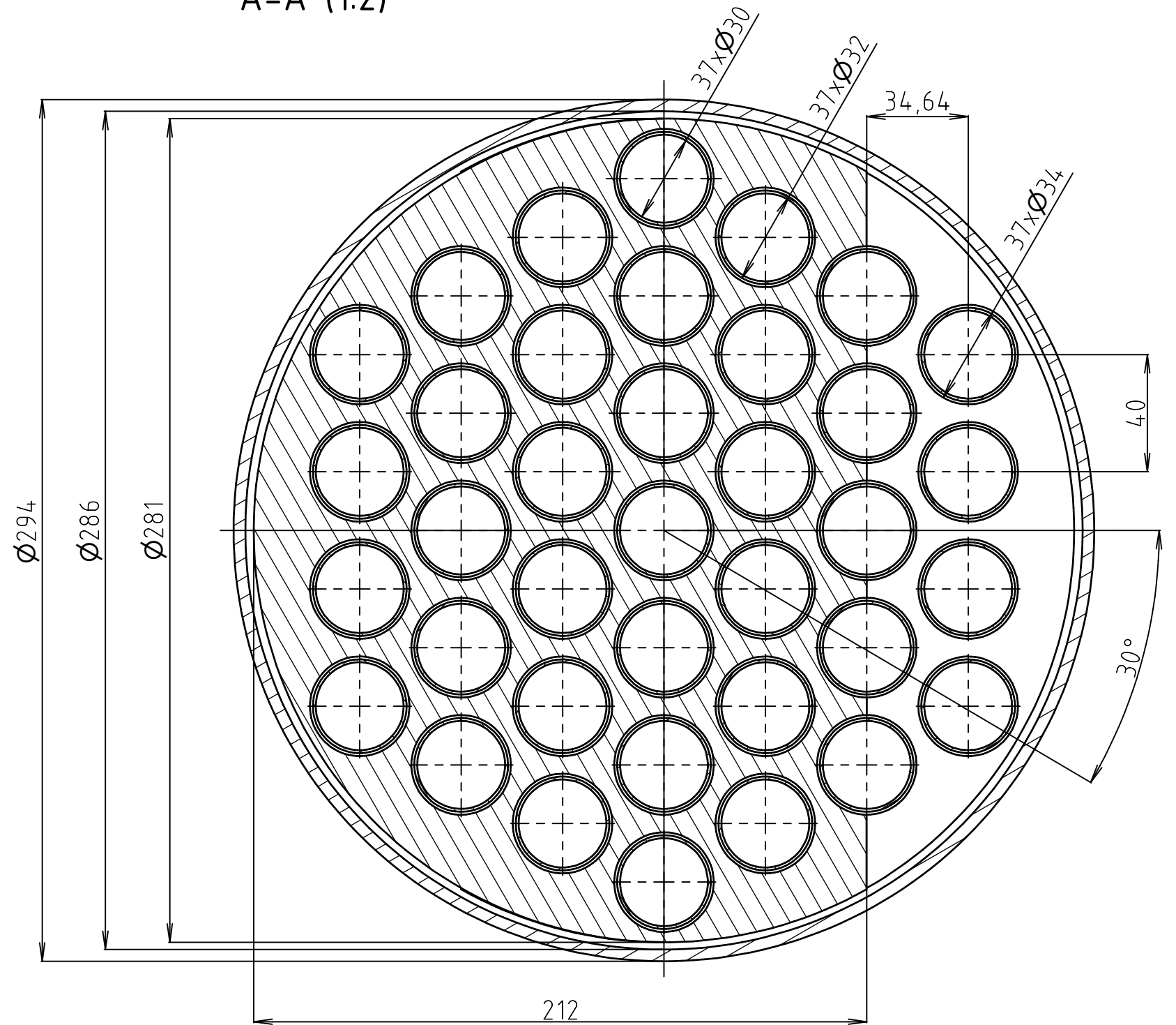
A-A (1:2)
