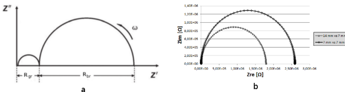
Obrázek 3: a) Teoretický průběh b) Simulovaný průběh impedanční charakteristiky.
