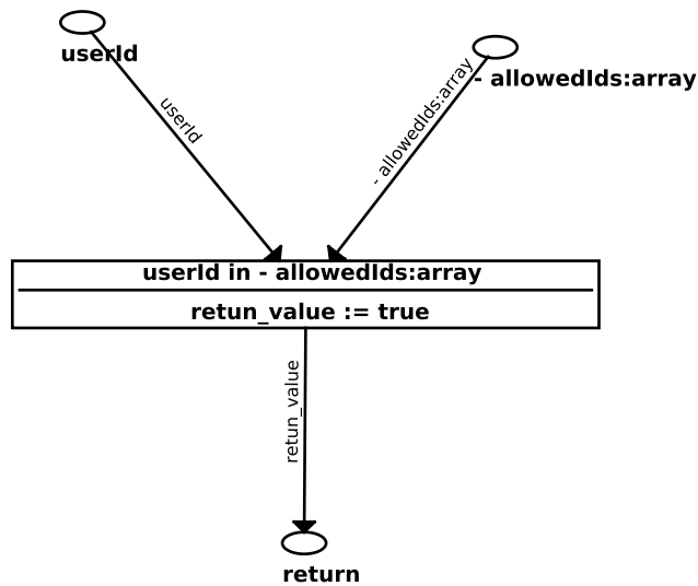
Obrázek 3.6: Metoda isUserAllowed popsána objektivě orientovanou Petriho sítí.
