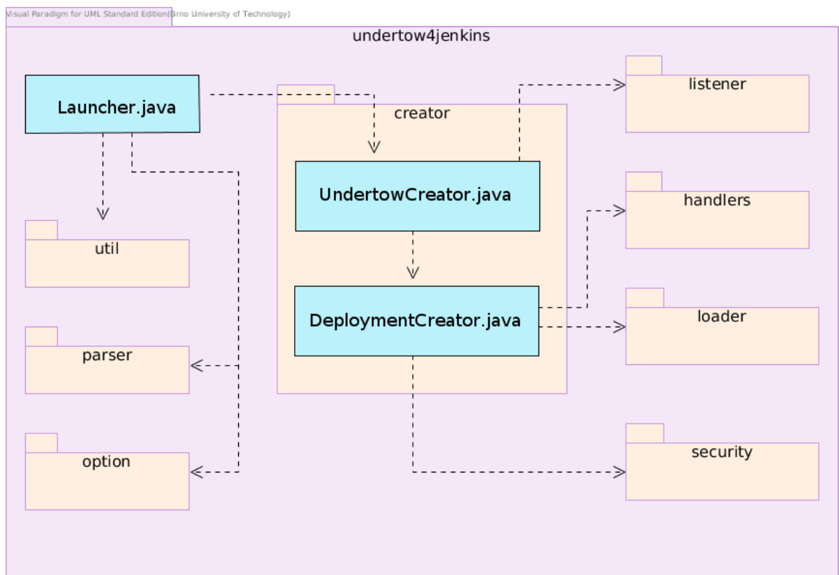
Obrázek 4.1: Diagram balíků zachycující architekturu vytvořeného servlet kontejneru rozšířený o tři nejdůležitější třídy
