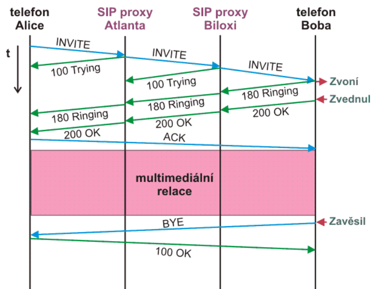
Obrázek 1.2 Ukázka SIP transakce, (dostupný z WWW: http://upload.wikimedia.org/wikipedia/cs/4/4c/SIP.png )
