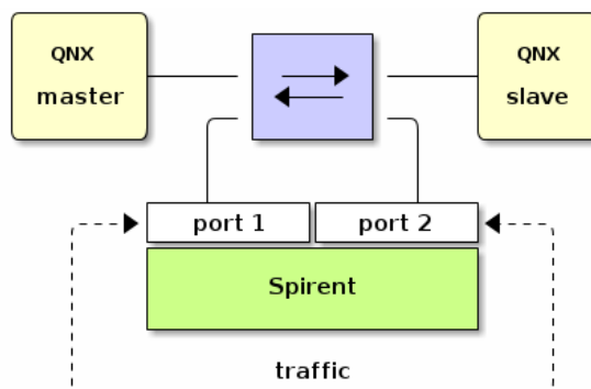
Obrázek 6.8: Schéma zapojení
