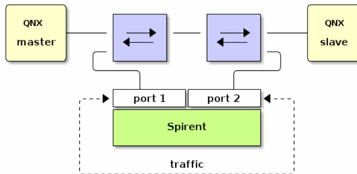
Obrázek 6.21: Schéma zapojení
