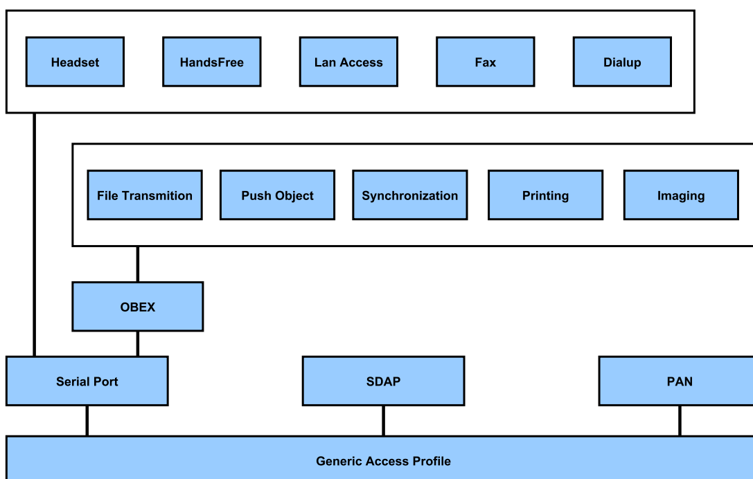
Obrázek 2.4: Hierarchie profilů. [24]
